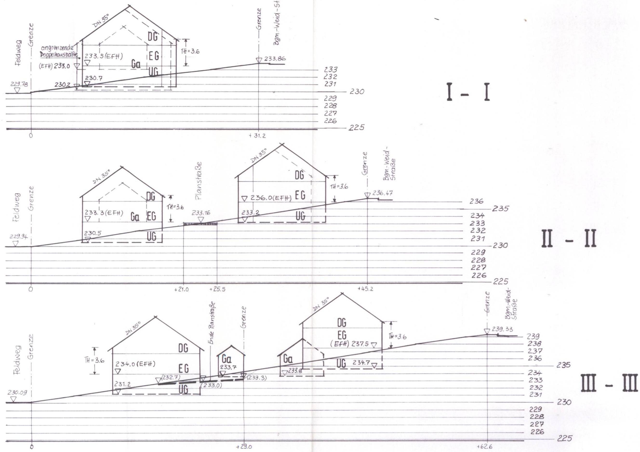
SYSTEMSCHNITTE M. 1: 250
